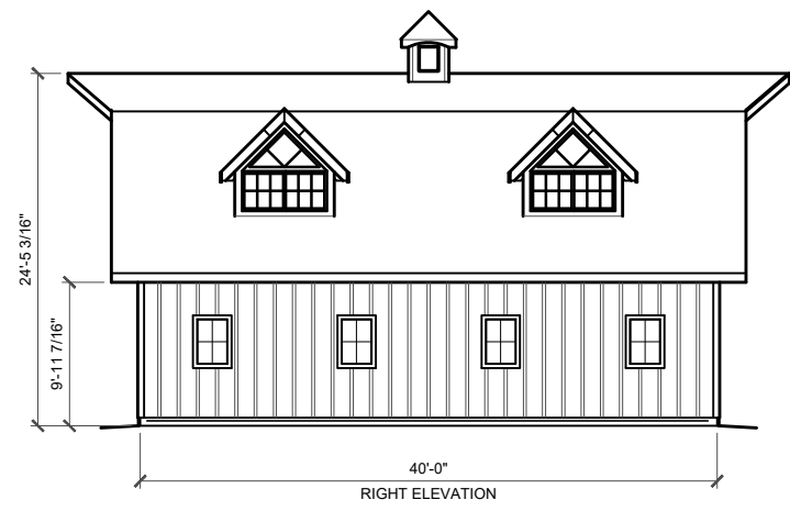
RIGHT ELEVATION
